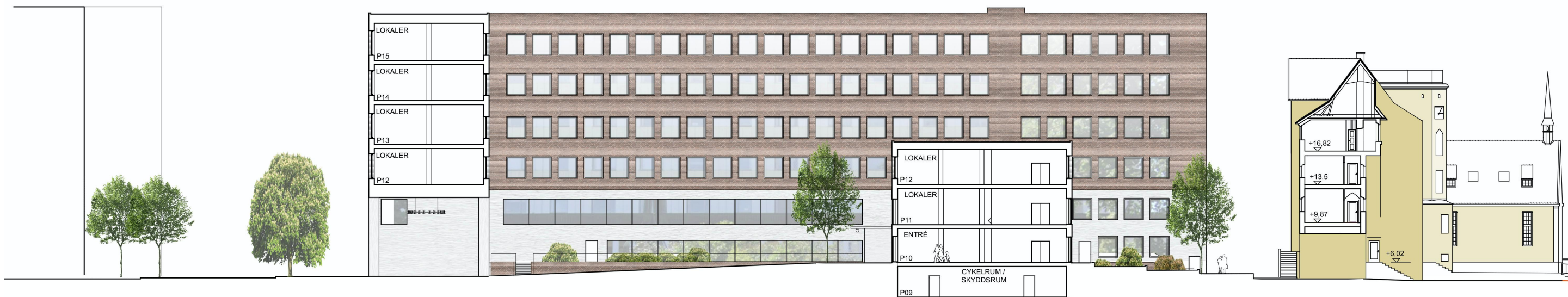
FASAD MOT GÅRDEN / SEKTION
